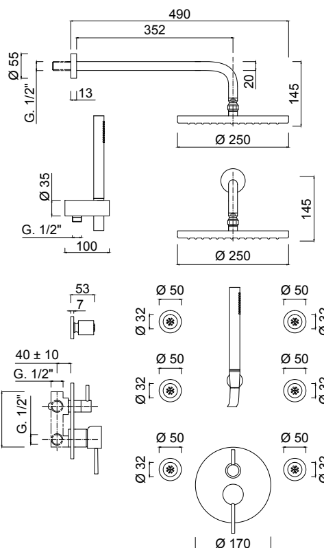
Soffione tondo D.250 mm Round showerhead Ø 250 mm
